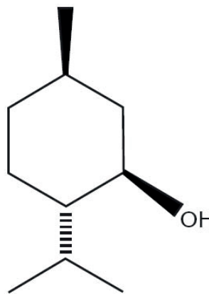
Fig. 1. Formula desarrollada del mentol
